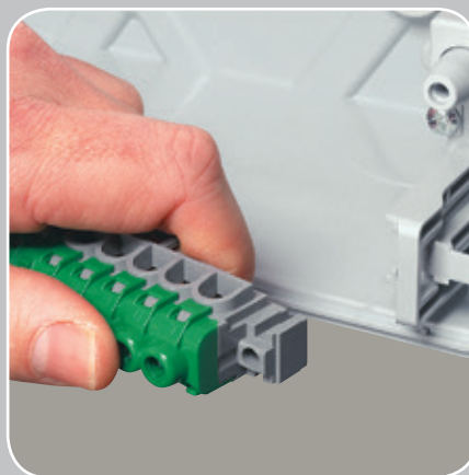
▲ Bornier extractible et repositionnable facilement, en partie haute et basse du coffret
