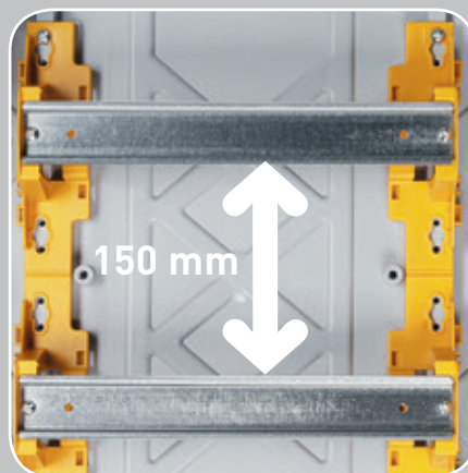
▲ Espace entre rails (permettant d'utiliser le peigne vertical)
