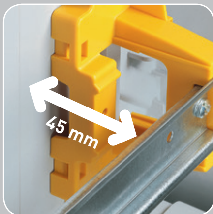
▲ Espace sous-rails (rail 2 positions ajustable en profondeur)
